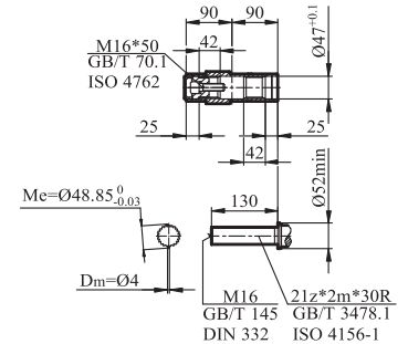
GKV/GKVZ/GKVF67输出轴
