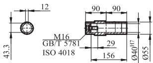
GKA/GKAZ/GKAF67输出轴
