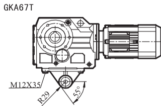
GKA/GKAZ/GKAF67输出轴
